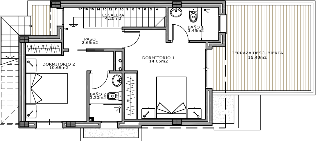
PLANTA PRIMERA
