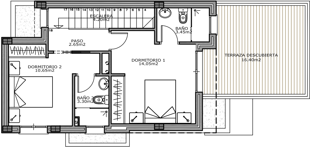
PLANTA PRIMERA
