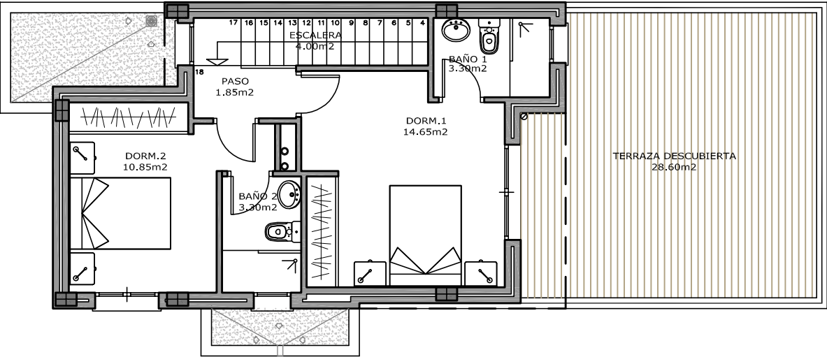
PLANTA PRIMERA
