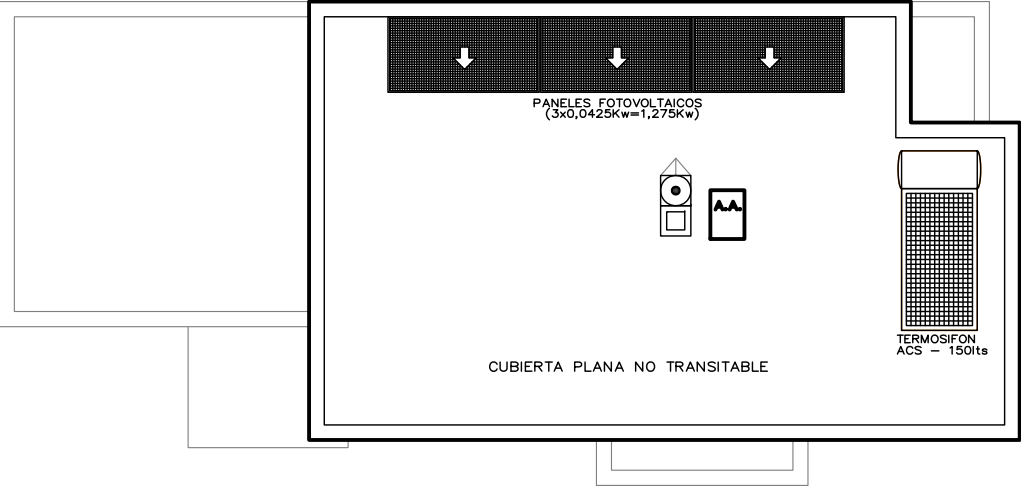
PLANTA CUBIERTAS
