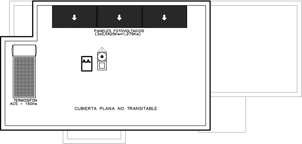
PLANTA CUBIERTAS
