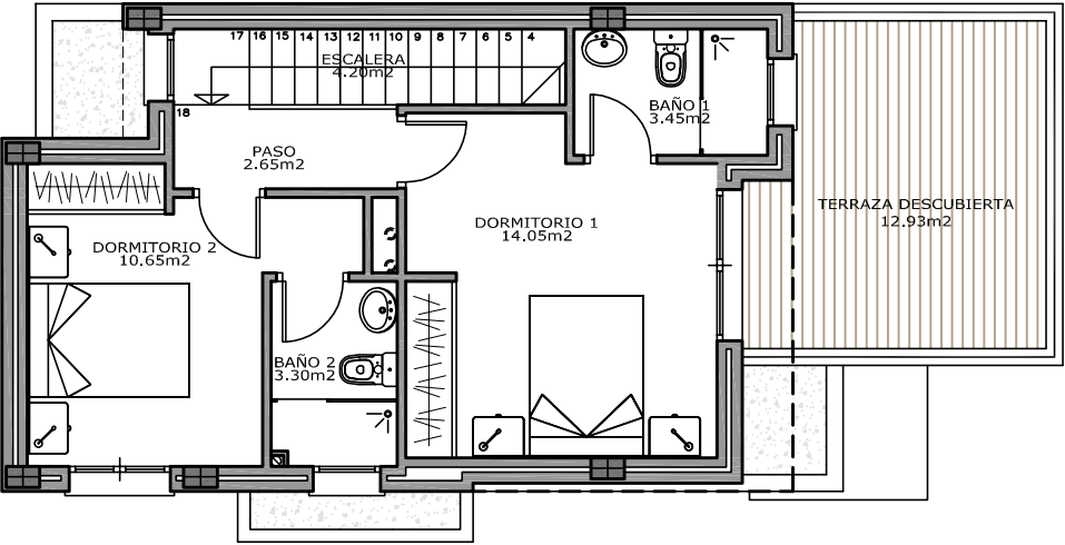
PLANTA PRIMERA
