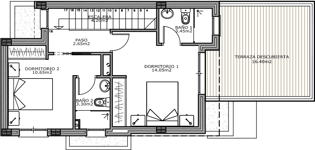
PLANTA PRIMERA
