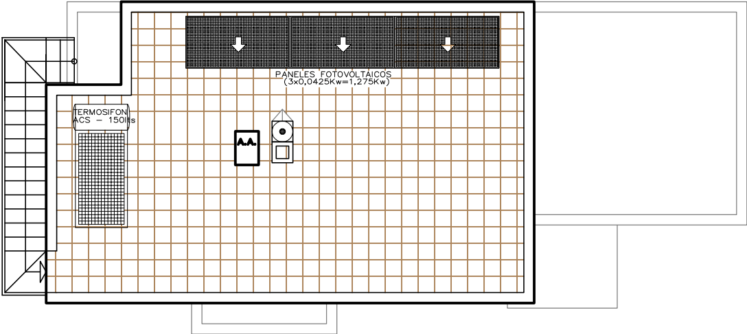
PLANTA CUBIERTAS
