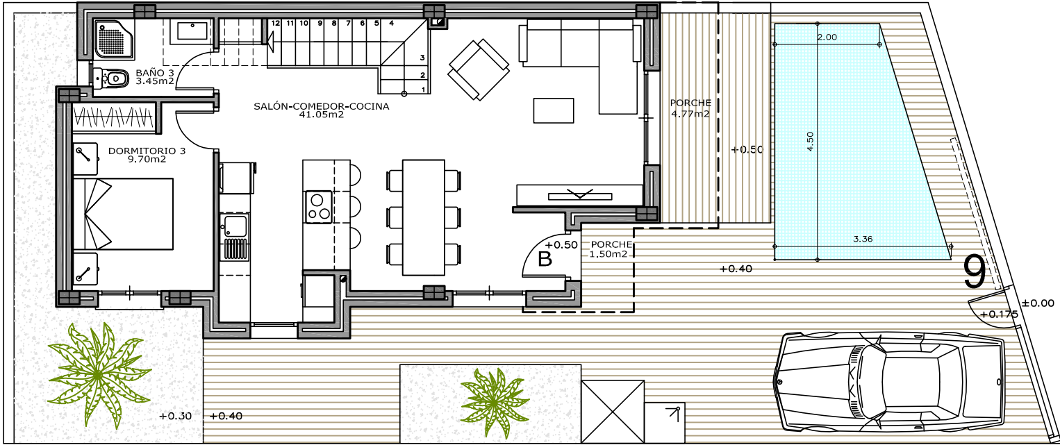
PLANTA BAJA
