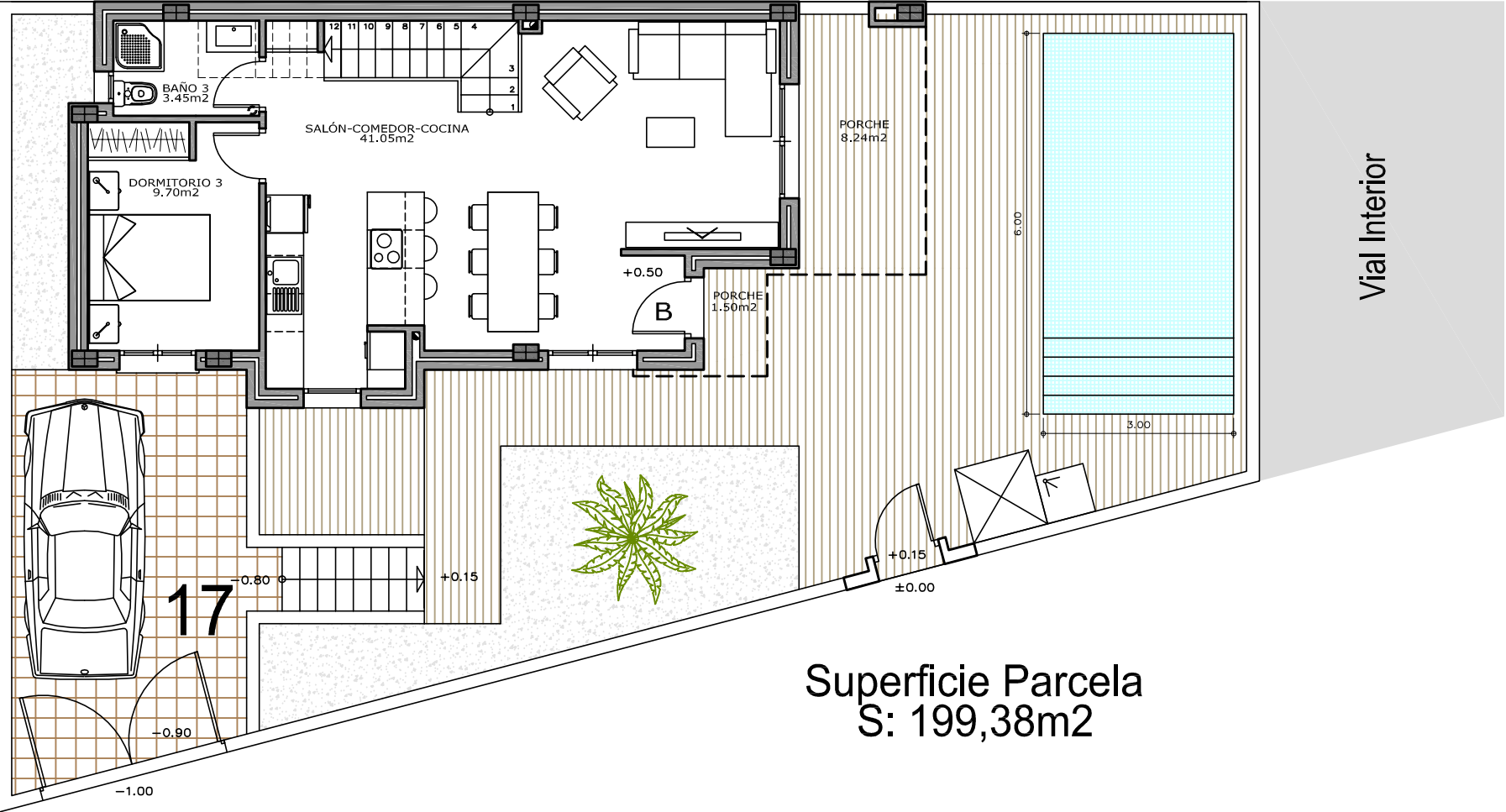
PLANTA BAJA
