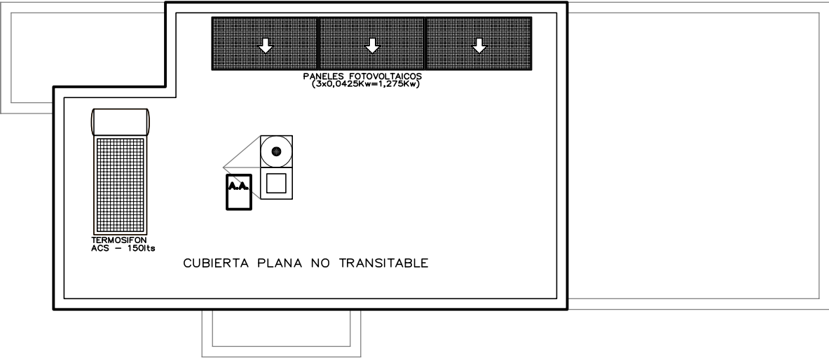
PLANTA CUBIERTAS
