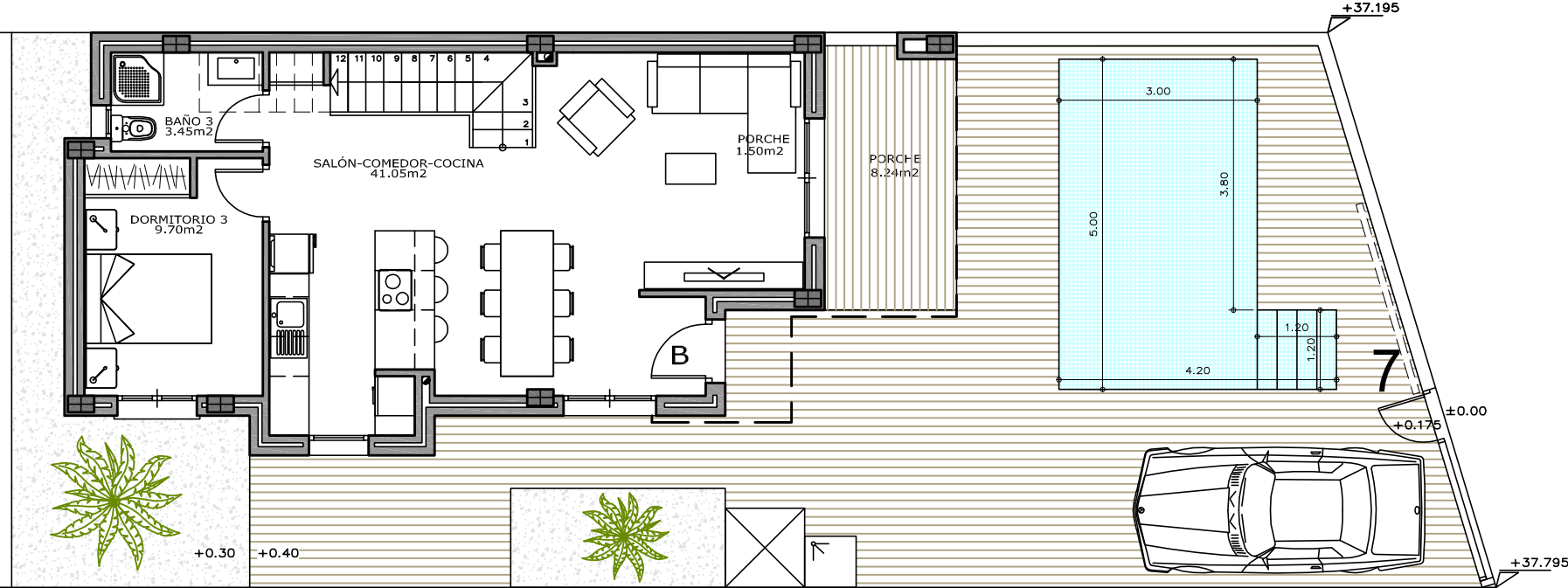
PLANTA BAJA
