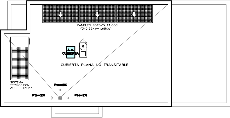
PLANTA CUBIERTAS
